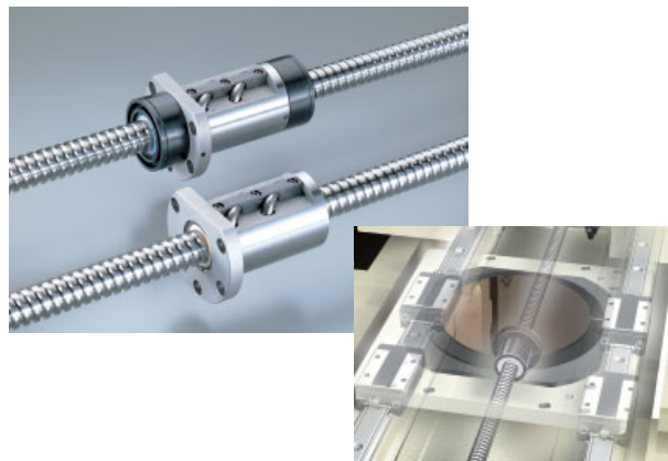
半導体製造装置 (ダイシングソー) での使用例
